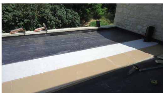
Pose de la première couche de laies d'étanchéité bitumeuse (rouleau bitume élastomère)
