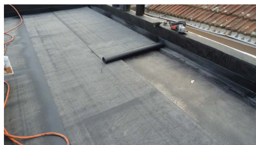
Pose de la seconde couche de protection
